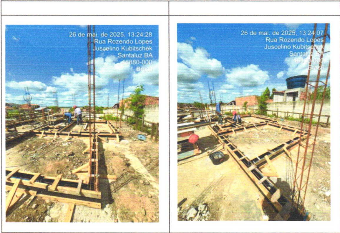
AMARRAÇÃO DE VIGAS E PILARES
