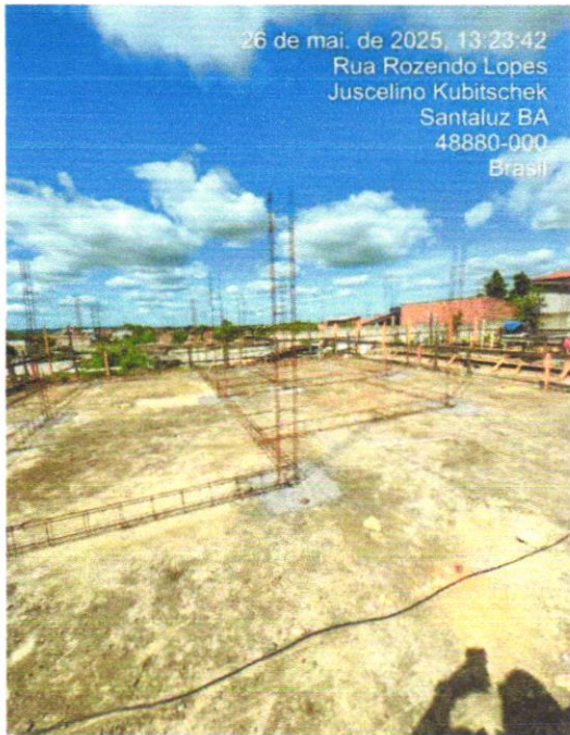
AMARRAÇÃO DE VIGAS E PILARES
